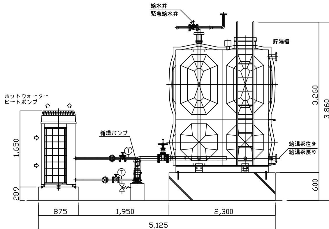
立面図 1:50
