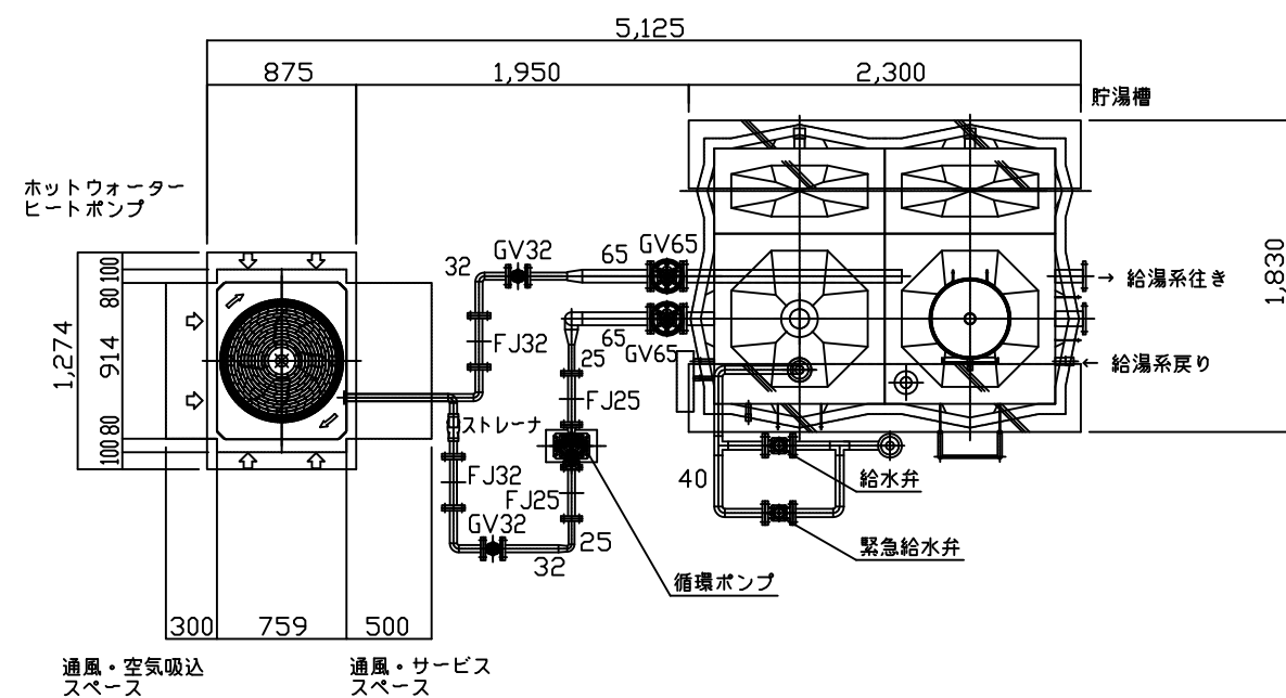
平面図 1:50
