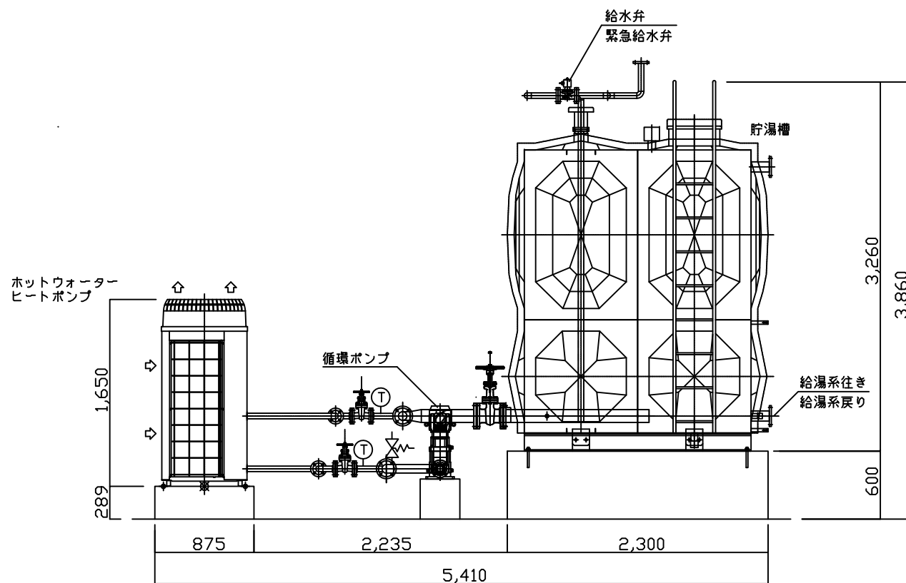
立面図 1:50
