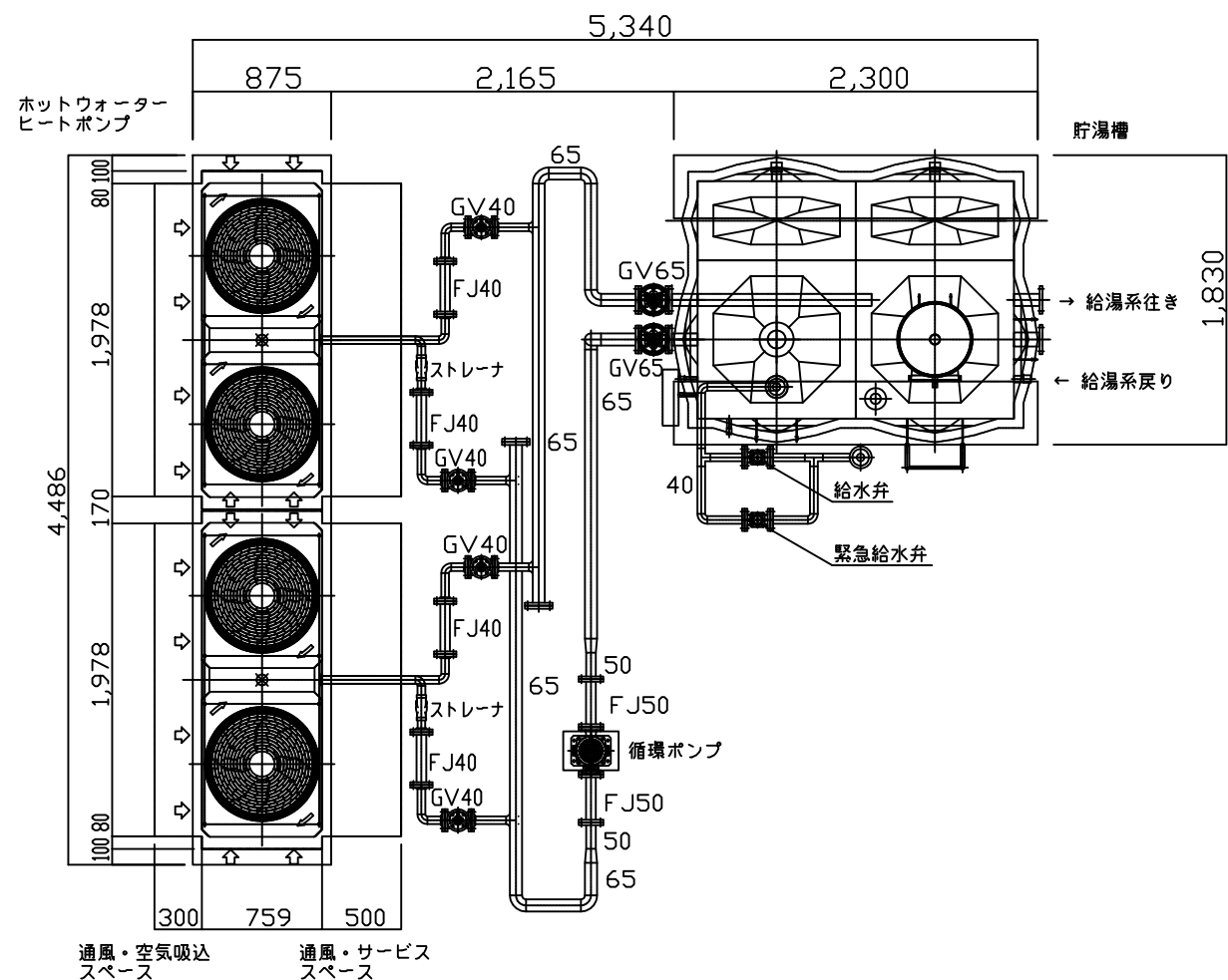
平面図 1:50
