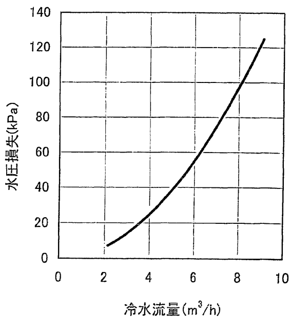
冷却器水圧損失
