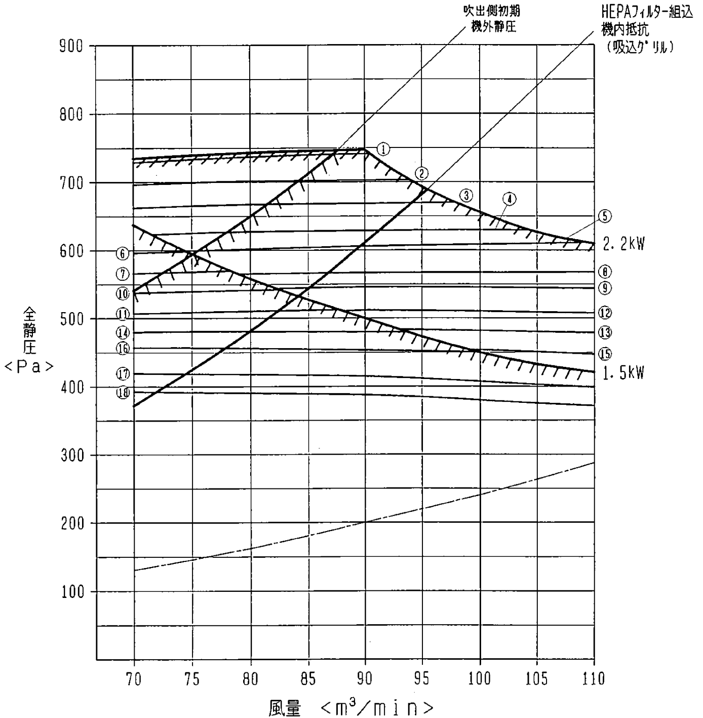
送風機性能線図
