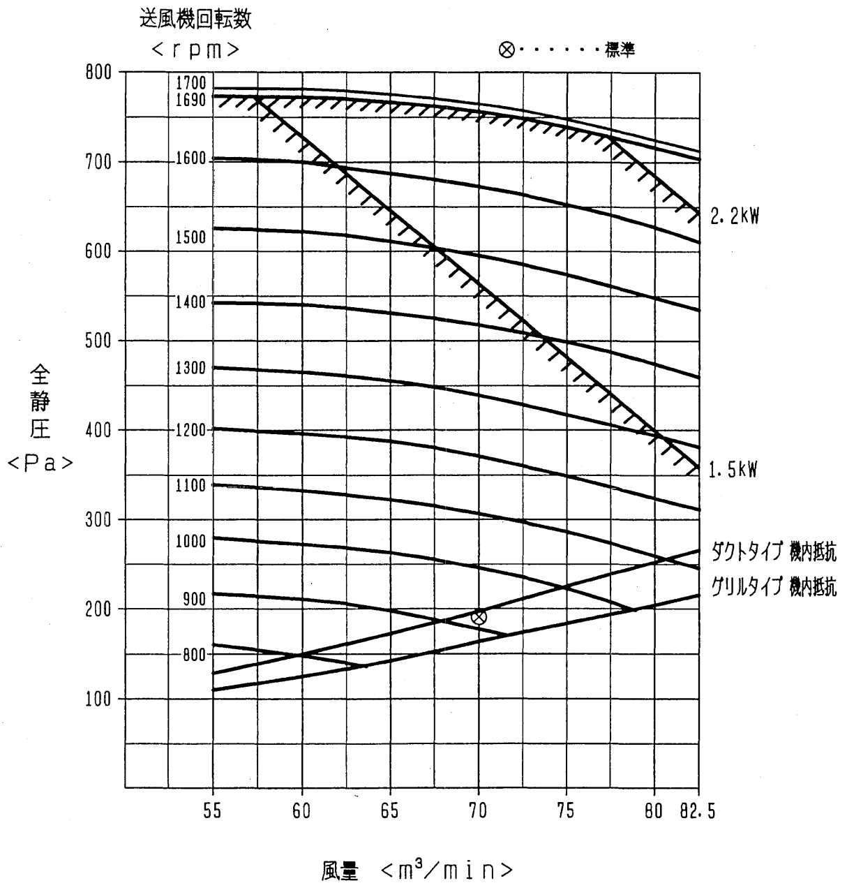
送風機性能線図
