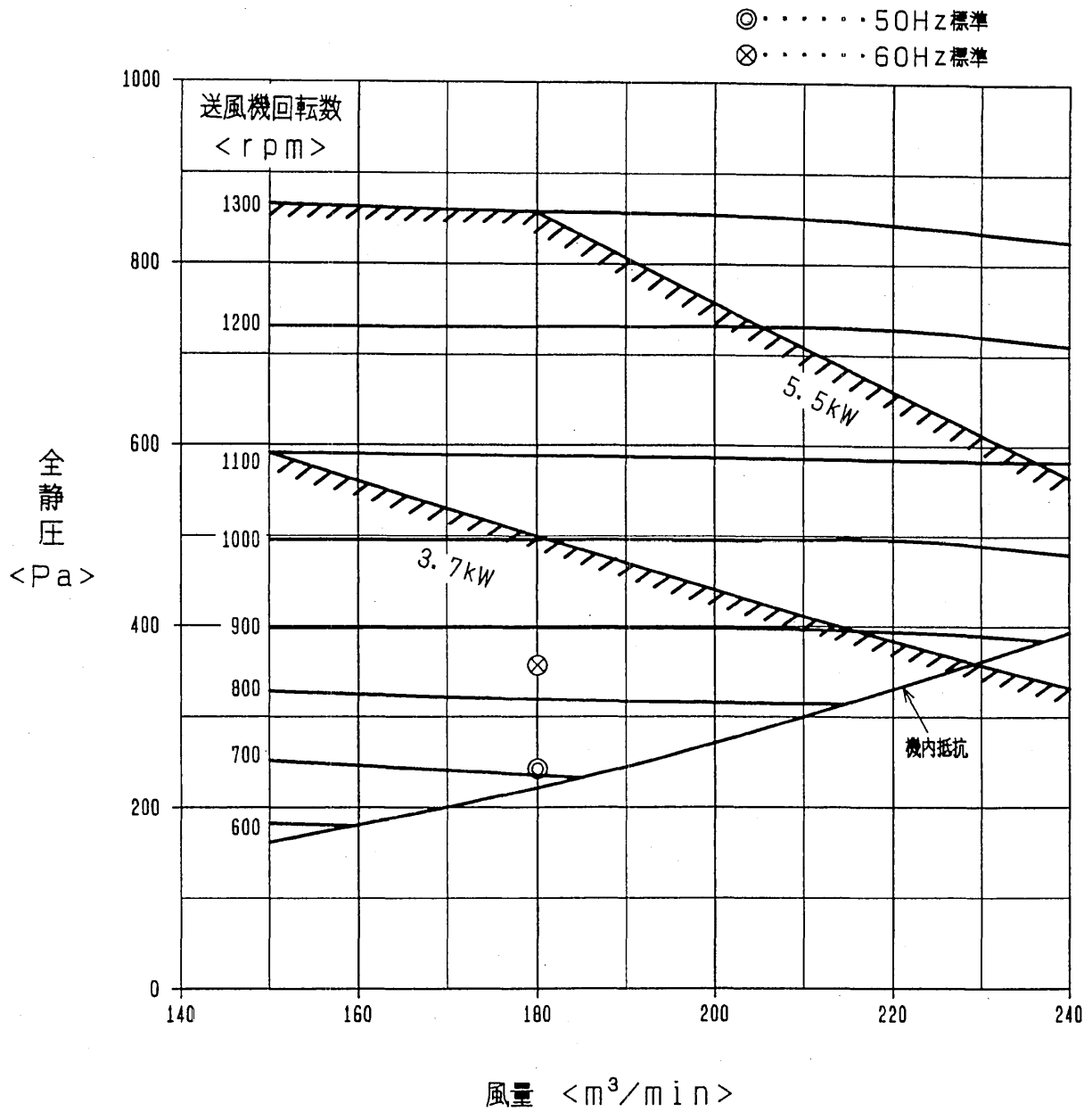
送風機性能線図
