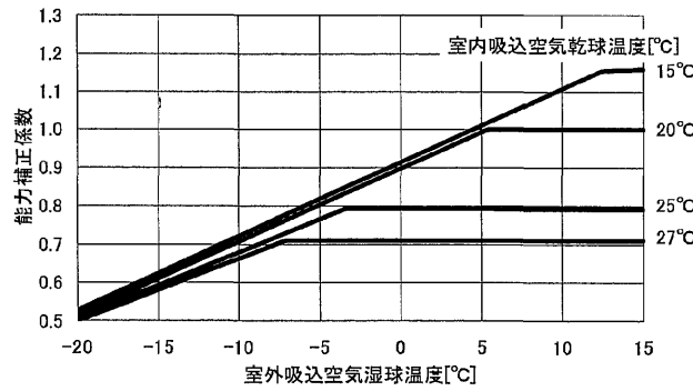
③暖房温度補正
