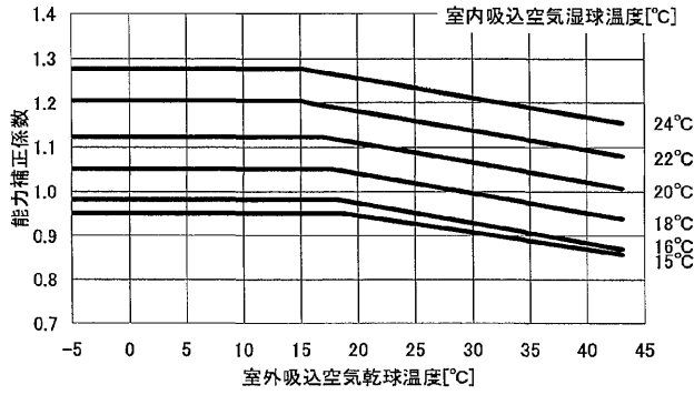
①冷房温度補正
