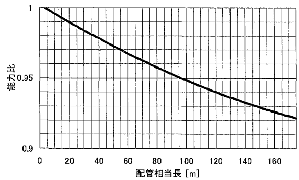
④暖房配管長補正
