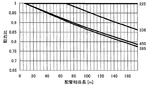
②冷房配管長補正
