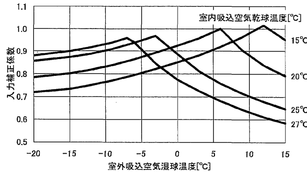
⑤霜取補正
