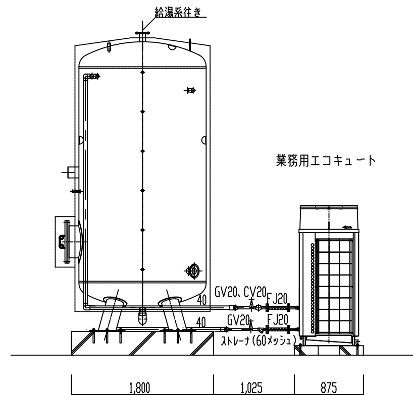
背面図 1:50
