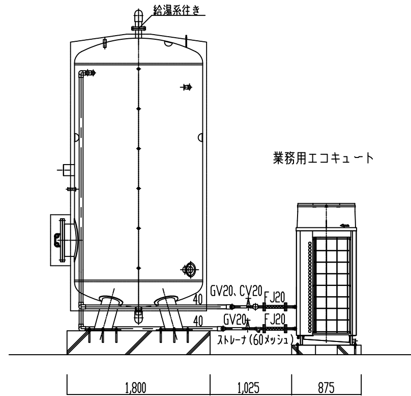
背面図 1:50
