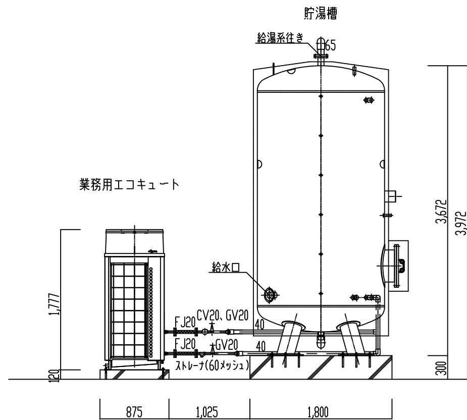
正面図 1:50
