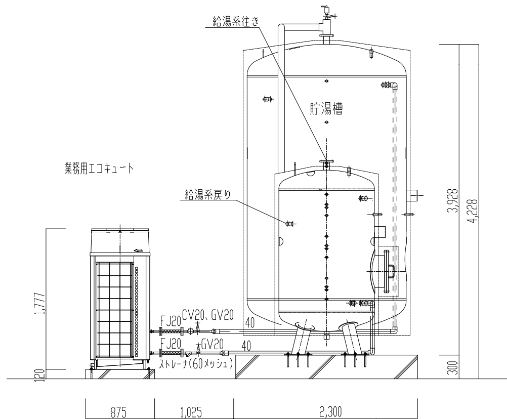
正面図 1:50
