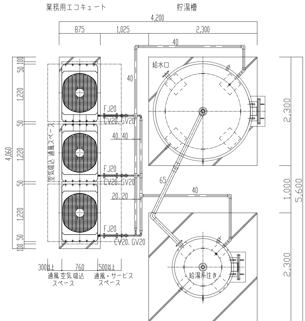
平面図 1:50
