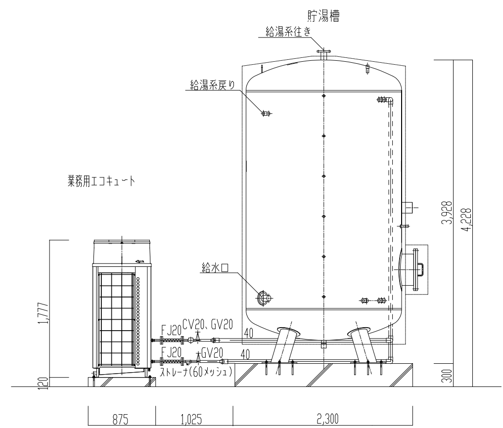
平面図 1:50
