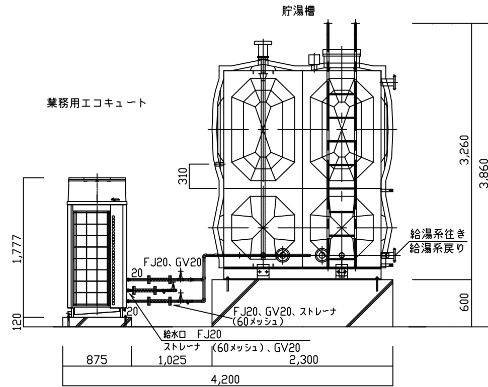
立面図 1:50
