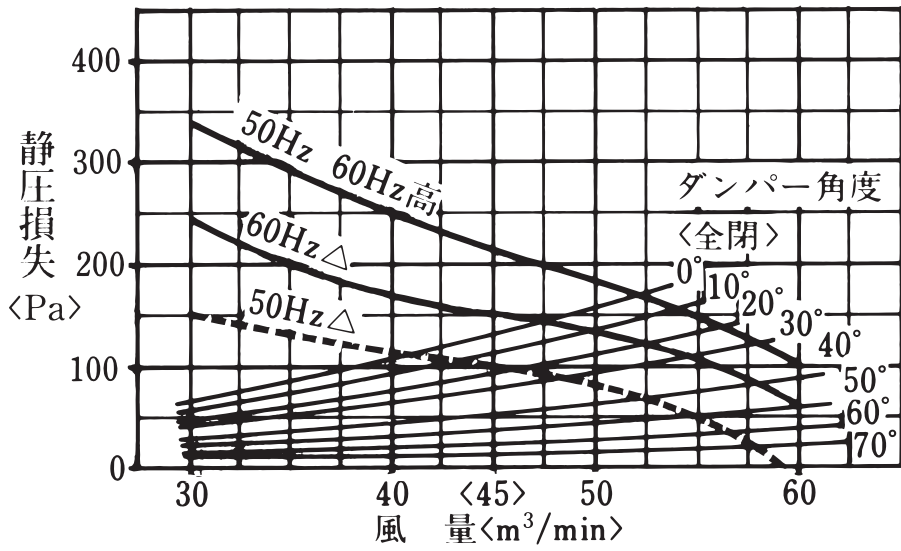
<ダクトタイプ増加圧損>
