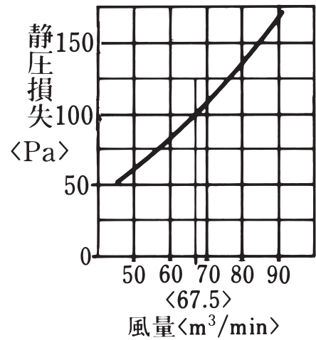
<ダクトタイプ増加圧損>
