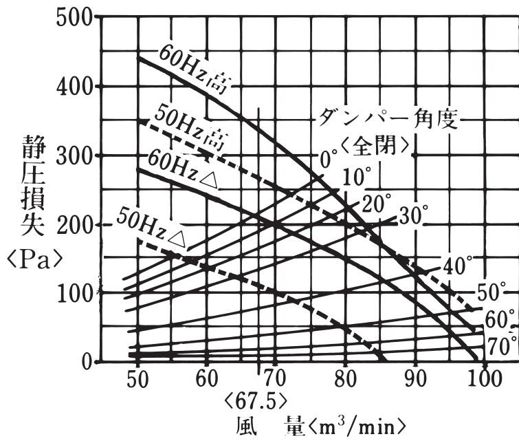
<ダクトタイプ増加圧損>
