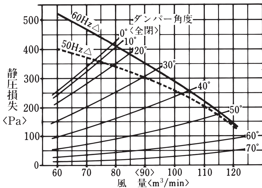
<ダクトタイプ増加圧損>
