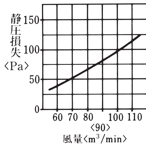
<ダクトタイプ増加圧損>
