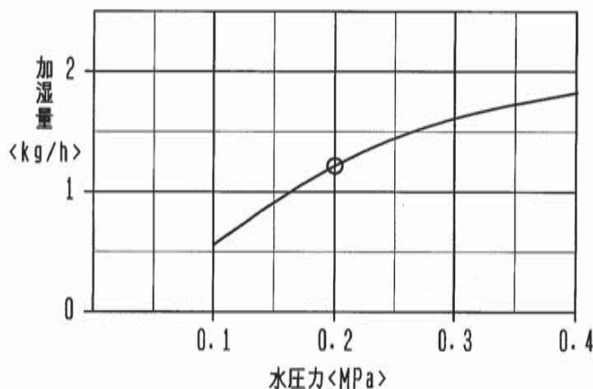
水スプレー式加湿器能力線図
