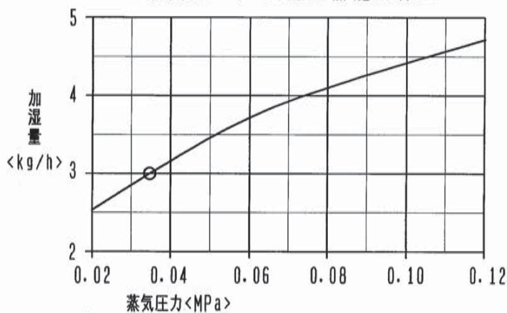
蒸気スプレー式加湿器能力線図
