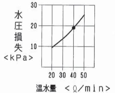
水圧損失線図
