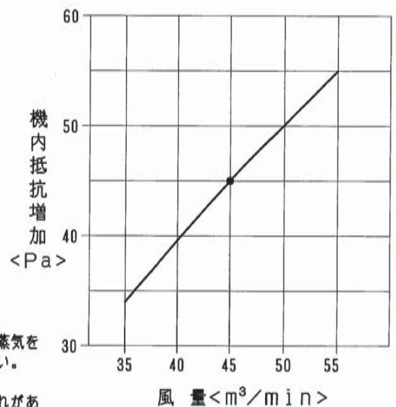
温水・蒸気加熱器機内抵抗線図<別売部品>
