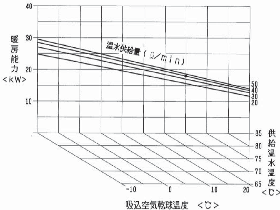
温水加熱器能力線図<別売部品>
