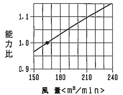
風量補正線図
