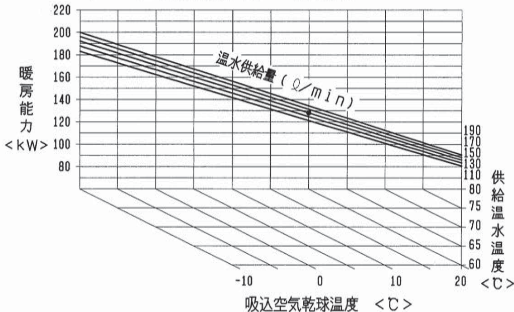
温水加熱器能力線図<別売部品>
