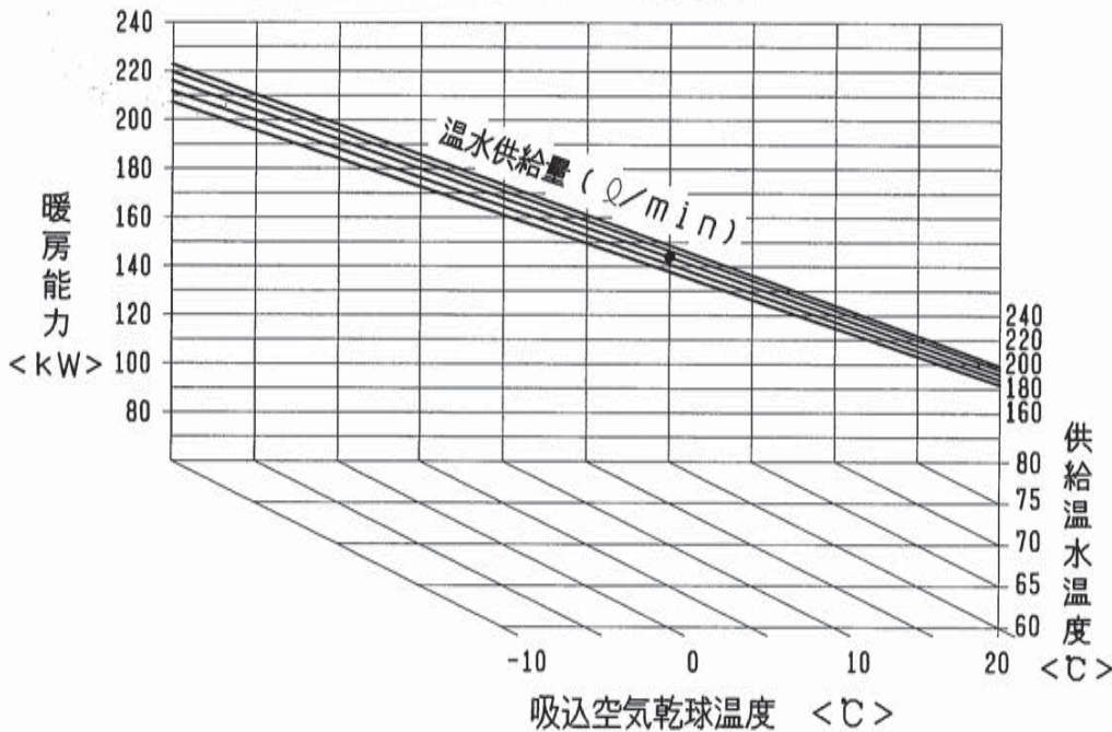
温水加熱器能力線図<別売部品>
