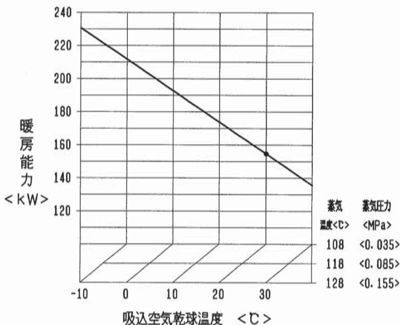
蒸気加熱器能力線図<別売部品>
