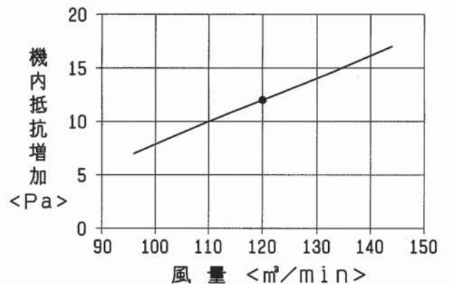
温水・蒸気加熱器機内抵抗線図<別売部品>
