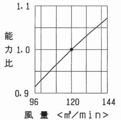
温水・蒸気加熱器 風量補正線図
