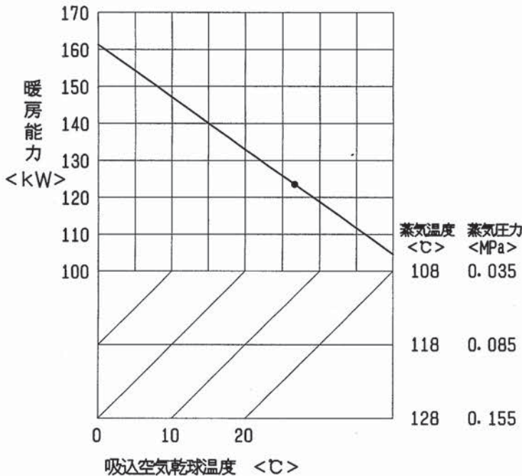
蒸気加熱器能力線図<別売部品>
