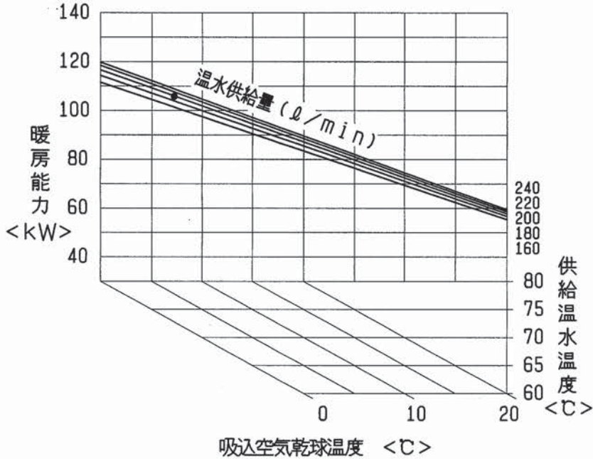
温水加熱器能力線図<別売部品>
