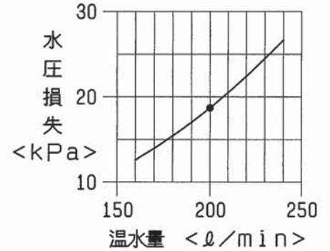
温水加熱器 水圧損失線図
