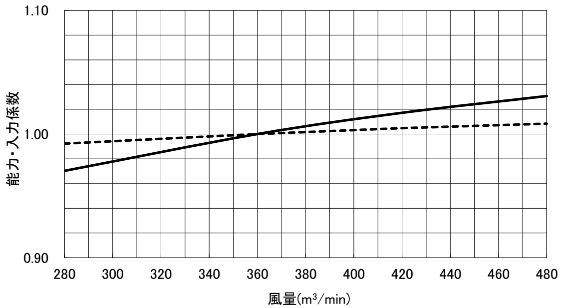
風量補正線図(床置、実線:能力、破線:入力) 【PFTV-P1120DM-E(1)】
