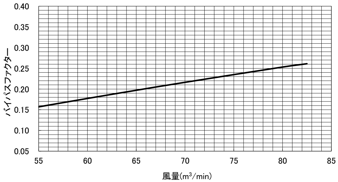
バイパスファクター線図 【PFTV-P224DM-E(1)】
