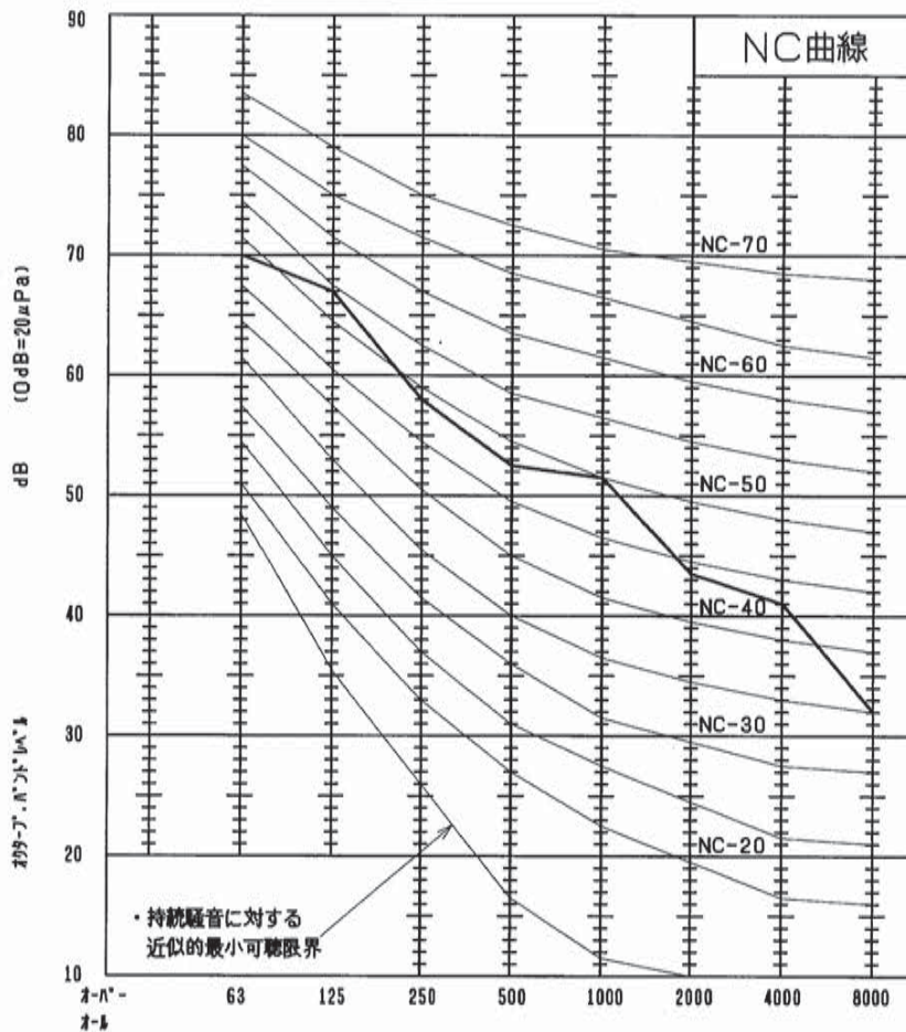
・オクターブバンド中心周波数Hz PFAV-P1000DM-E(1)-F 標準 パッケージエアコン騒音分析成績書<50/60Hz>
