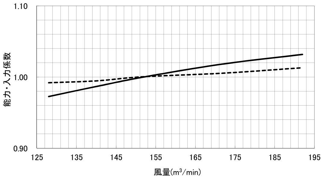
風量補正線図(実線:能力、破線:入力) 【PCHVD-P560DM-E(1)】 ●冷房
