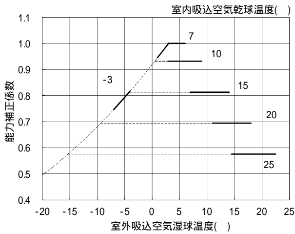
・暖房能力補正線図
