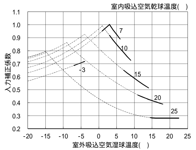
・暖房入力補正線図
