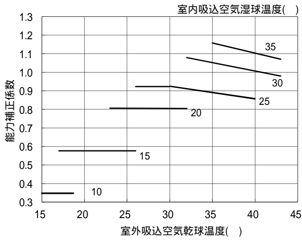
・冷房能力補正線図
