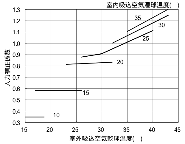
・冷房入力補正線図
