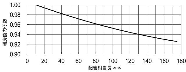
(3) P1120形
