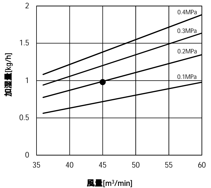
・PFAV-P335(V)DMJ1-F
