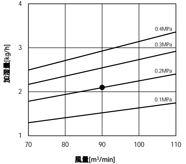
・PFAV-P280(V)DMJ1
