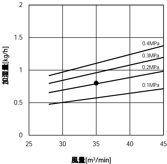
・PFAV-P265(V)DMJ1-F
