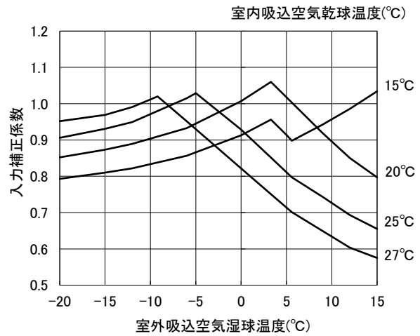
・暖房入力線図
