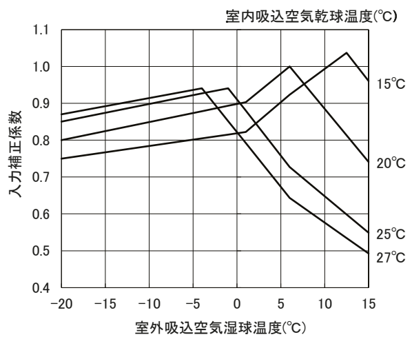
・暖房入力線図
