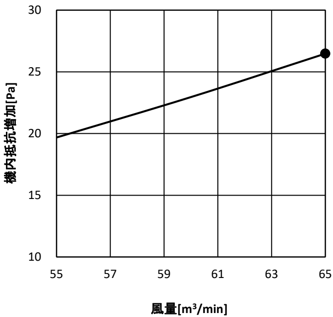
・PFAV-P224DME3
