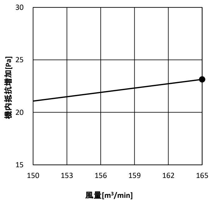
・PFAV-P560DME3
