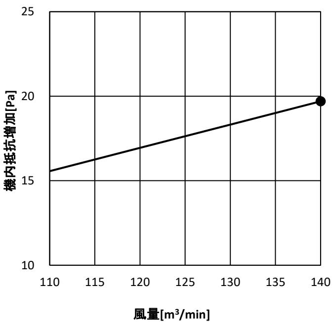
・PFAV-P450DME3
