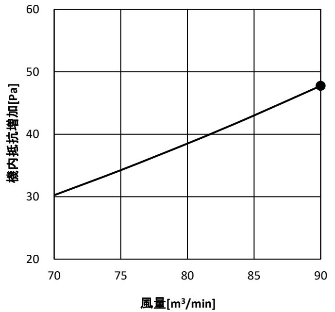
・PFAV-P280DME3
