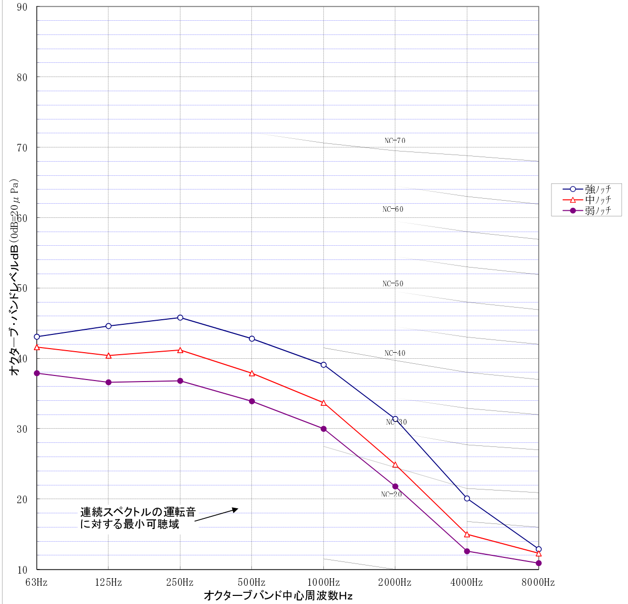
NC 曲線
