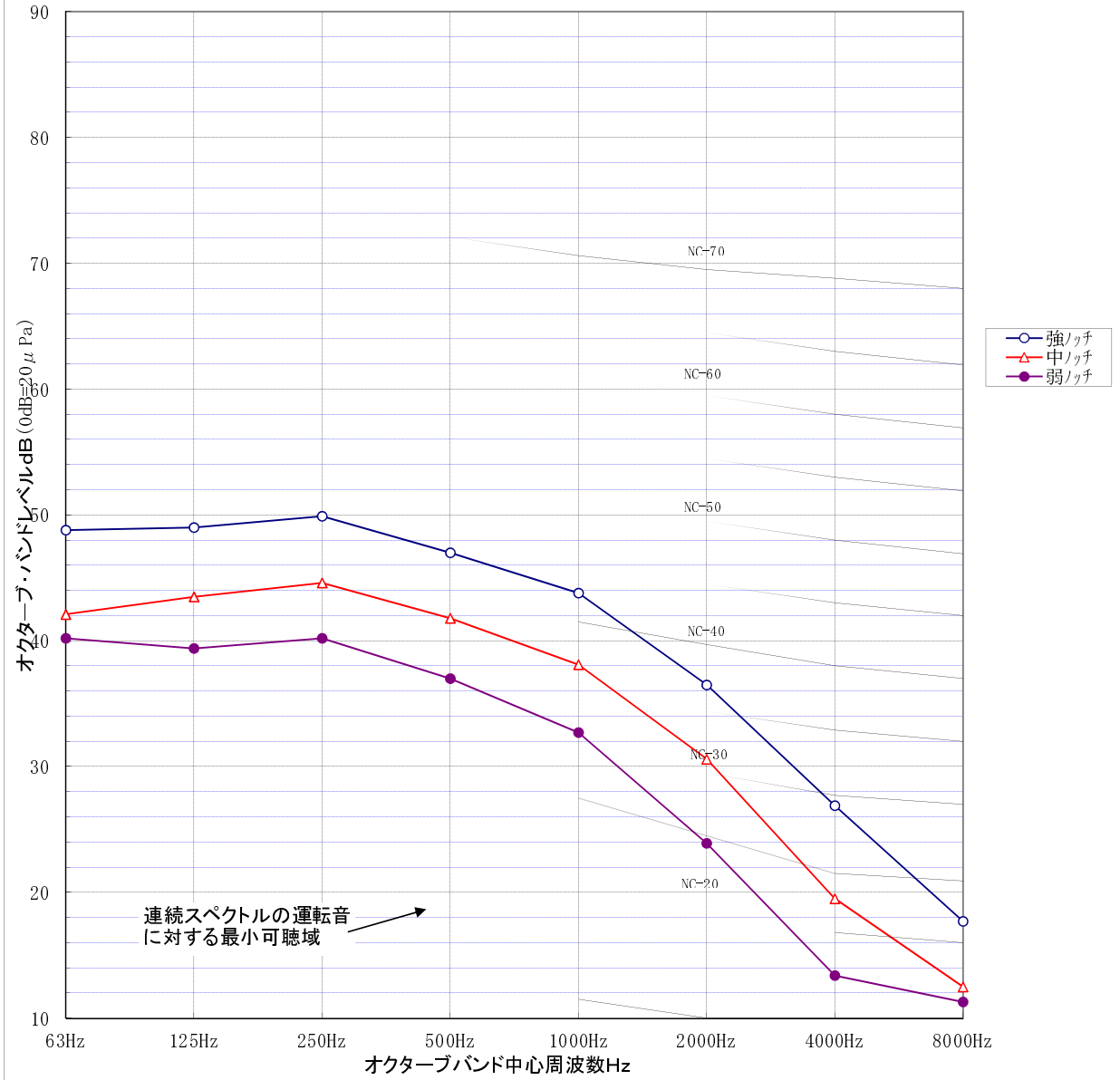
NC 曲線
