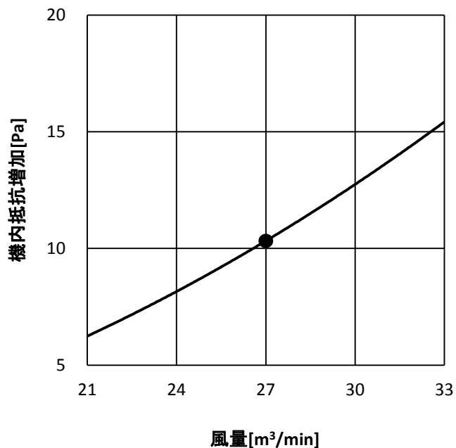
・PFAV-P80DMJ1
