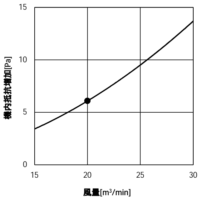
・PFAV-P167(V)DMJ1-F
