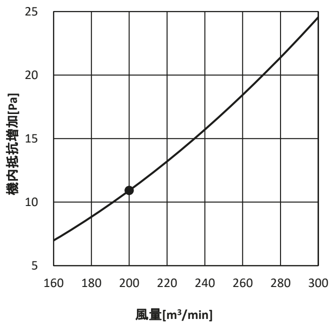
・PFAV-P1600DMJ3-F
