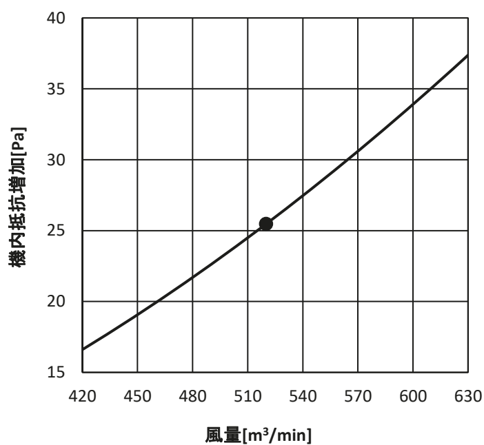
・PFAV-P1600DMJ3
