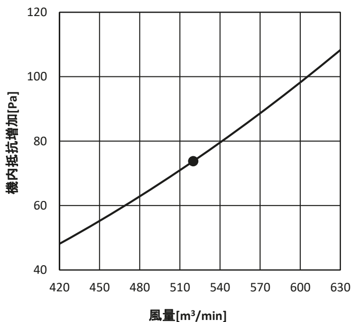
・PFAV-P1600DMJ3
