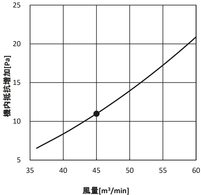
・PFAV-P335DMJ3-F
