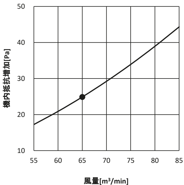
・PFAV-P224DMJ3
