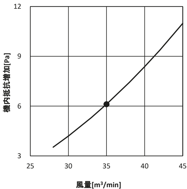
・PFAV-P265DMJ3-F
