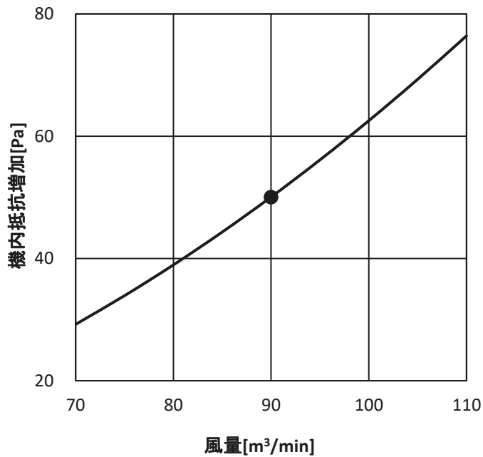
・PFAV-P280DMJ3
