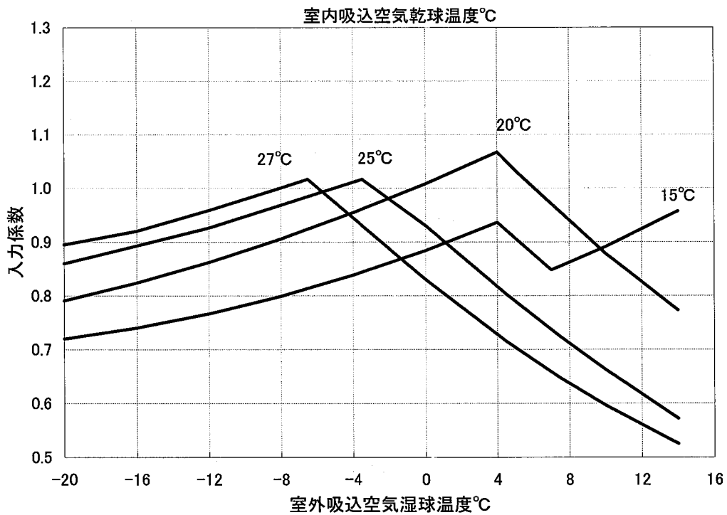
設備インバータ 霜取補正係数
