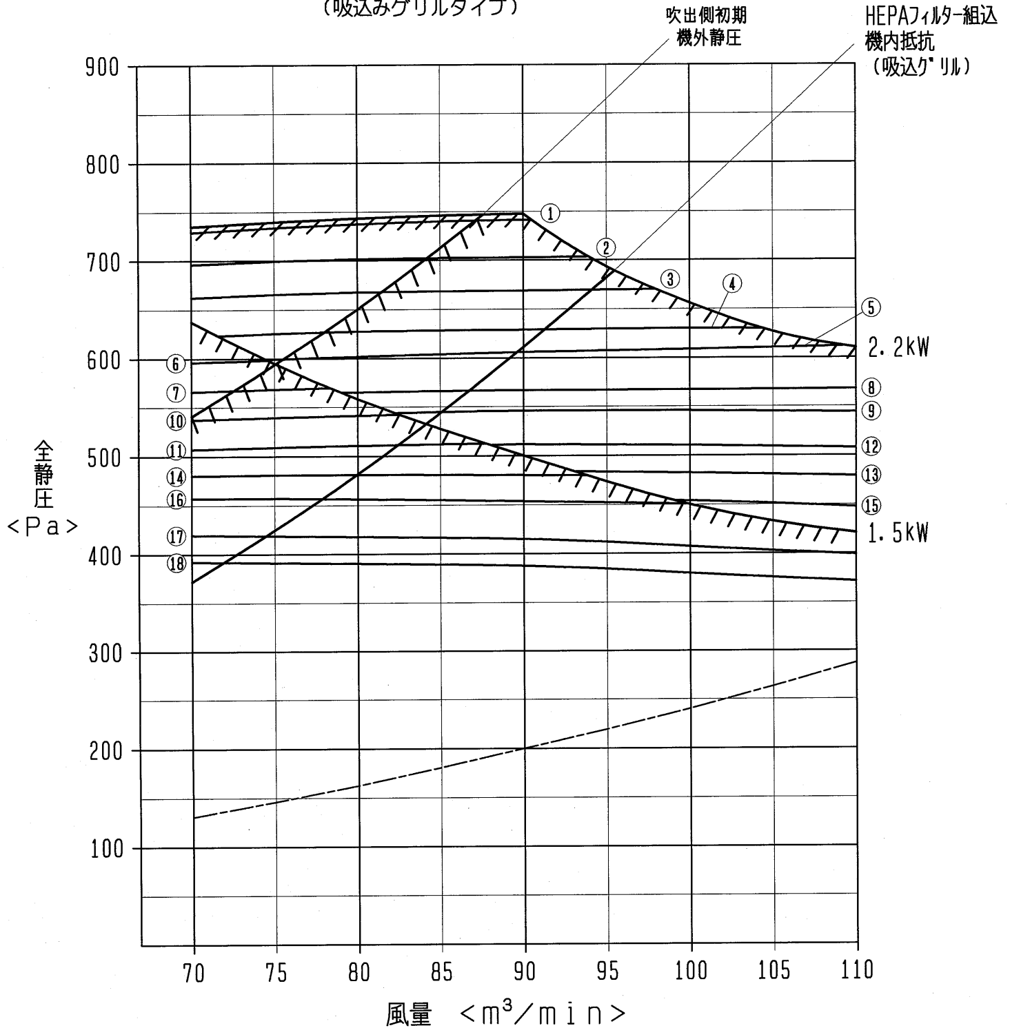
送風機性能線図
