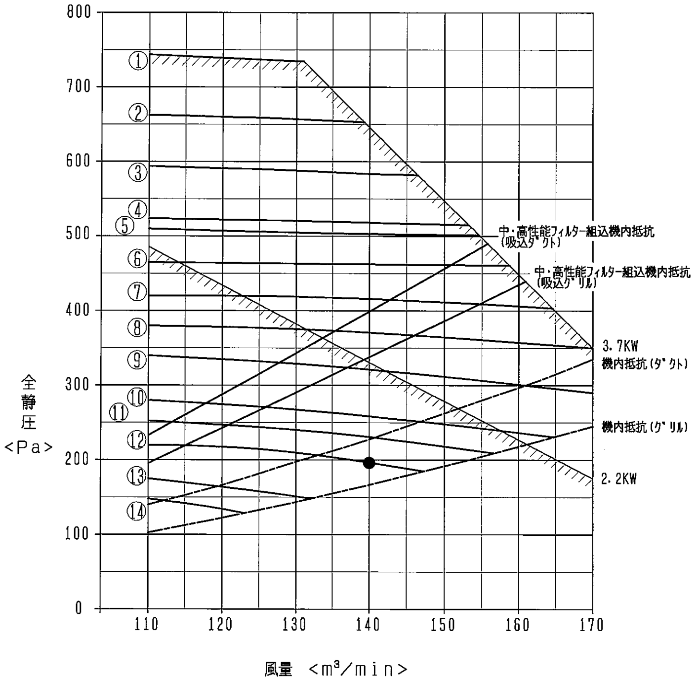
送風機性能線図
