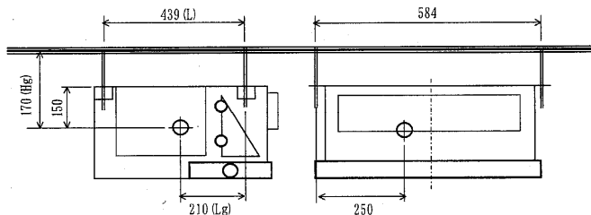
本図は左配管を示します(PEFY-P・ML)。右配管(PEFY-P・ML-R)は吹出口中央で対象となります。
