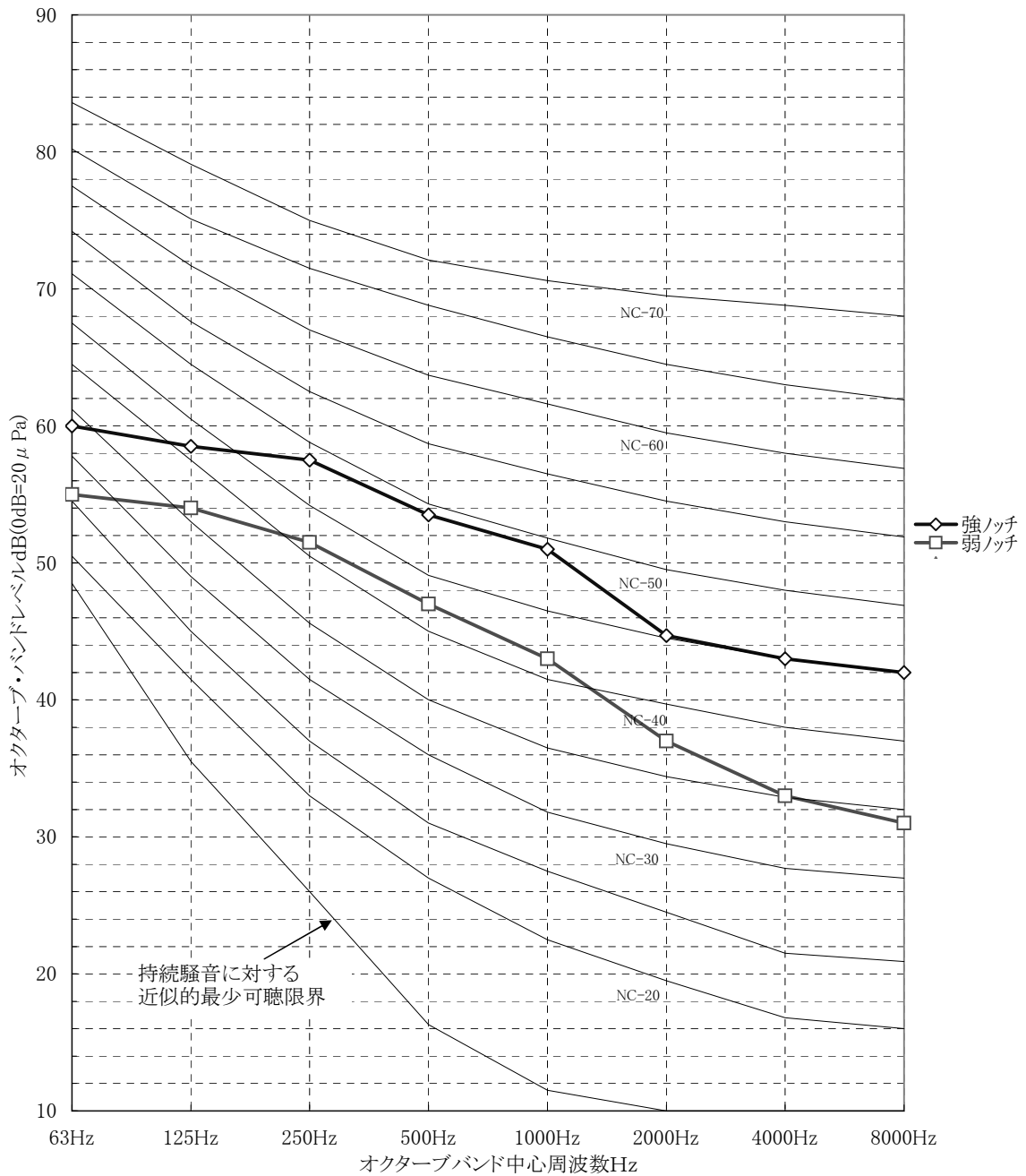
NC曲線
