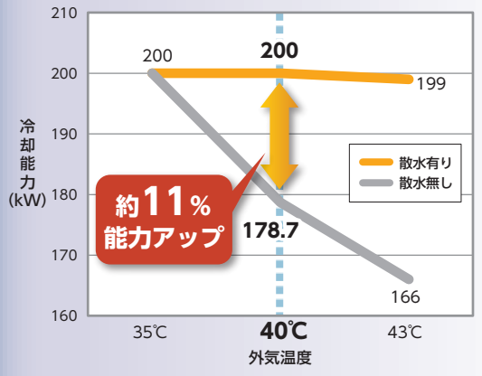
▶ 冷却能力比較 (冷房専用70HP、冷水出口水温7℃の場合)
