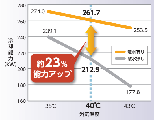
▶ 冷却能力比較 (冷房専用70HP、冷水出口水温15℃の場合)
