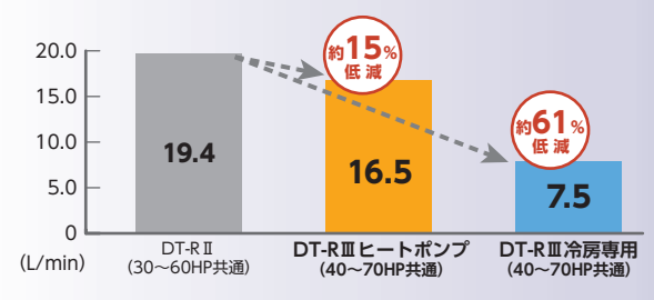
▶ 散水量比較 (80馬力・クールタフネス仕様60馬力は除く)
