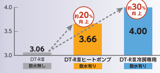
▶ COP比較 (70HP、外気温度35℃、冷水入口温度14℃、冷水出口温度7℃)
