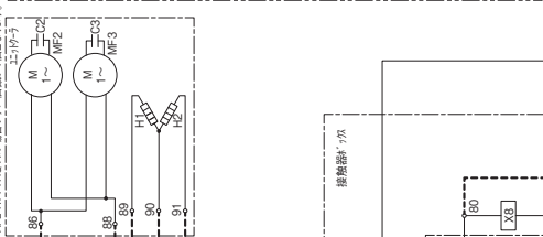
冷媒機内基板の詳細
