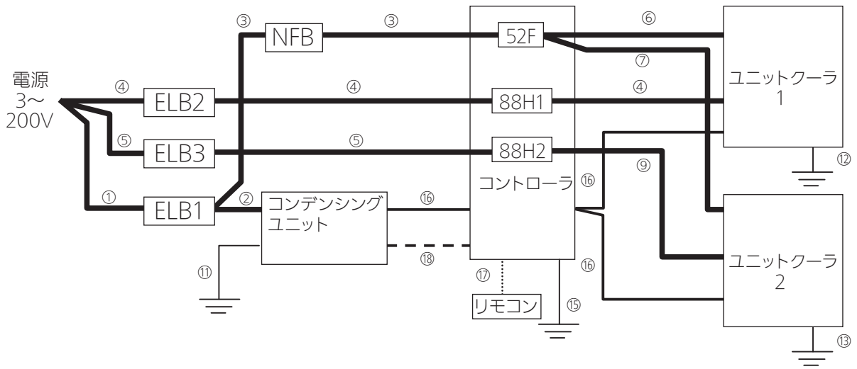
(2) ユニットクーラ 2 台接続の場合
