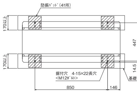
基礎寸法図 <横手方向の場合の穴(推奨)>
