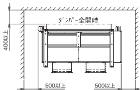
平面図
