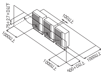
[4] 横連結で正面に障害物がある場合 (背面、側面、上方は開放)
