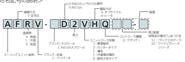
AFRVタイプ (仕様書はP.43、44に掲載)
