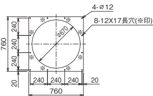
上面より見る
