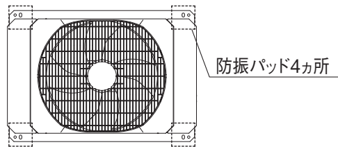
基礎寸法図 <奥行方向の場合の穴(推奨)>
