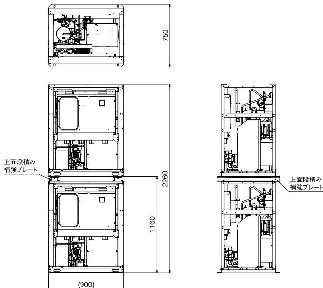
・DK-N45A使用時の組合せユニット寸法図
