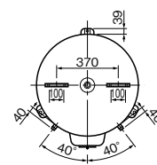
上面図
