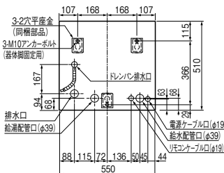
配管、アンカーボルト位置上面透視図 (SRG-201HD-B)
