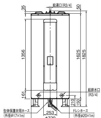
正面図
