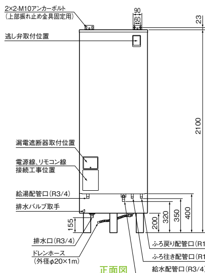
正面図
