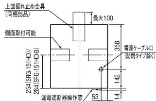
上面図
