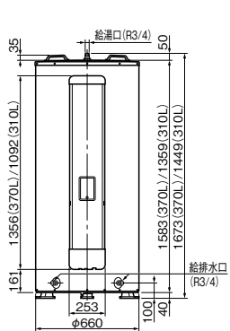
正面図
