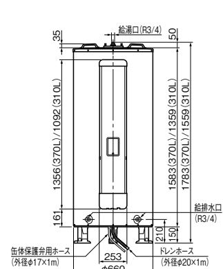
正面図
