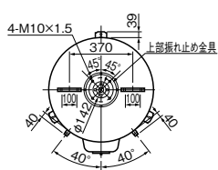
上面図
