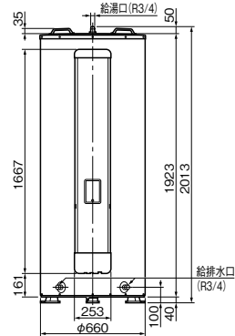
正面図
