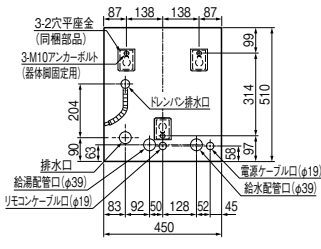
配管、アンカーボルト位置上面透視図 (SRG-151HD-B)
