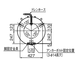
底面図
