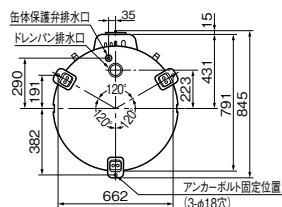
底面図
