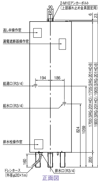
正面図
