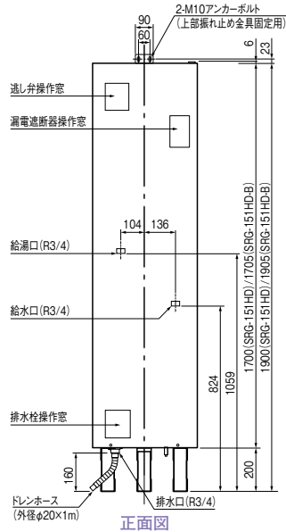
正面図
