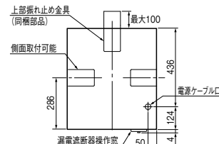
上面図
