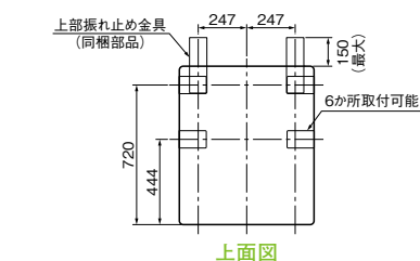
上面図
