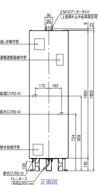
正面図
