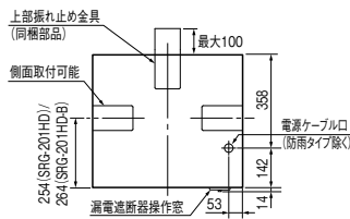
上面図
