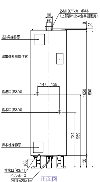
正面図
