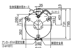
底面図
