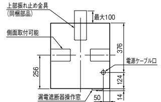
上面図
