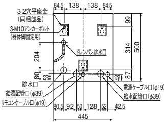
配管、アンカーボルト位置上面透視図 (SRG-151HD)
