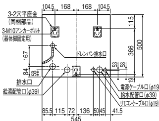
配管、アンカーボルト位置上面透視図 (SRG-201HD)
