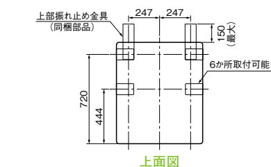
上面図
