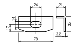
BWL型座金詳細図
