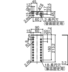
上部振れ止め金具 (同梱部品)
