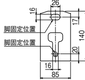
機体脚詳細図
