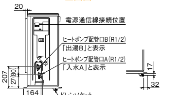
ドレンソケット取付位置側面図
