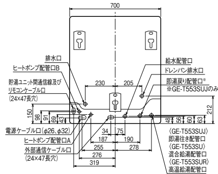
配管位置上面透視図
