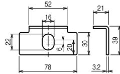
FWL型座金詳細図
