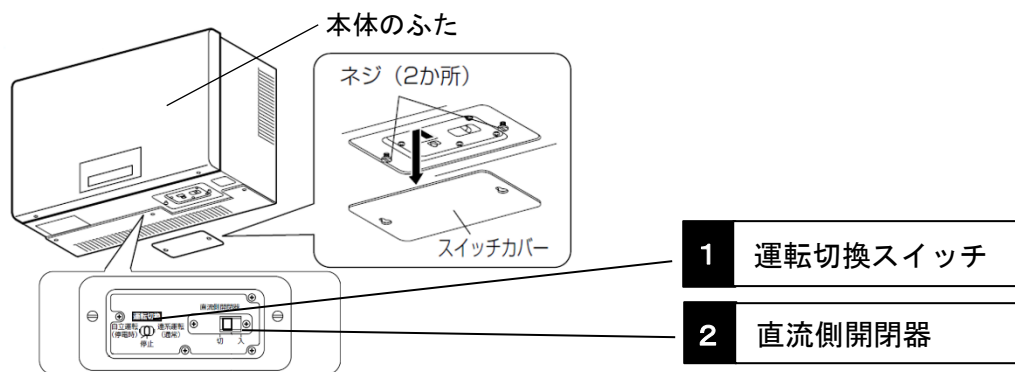
パワーコンディショナ操作部
